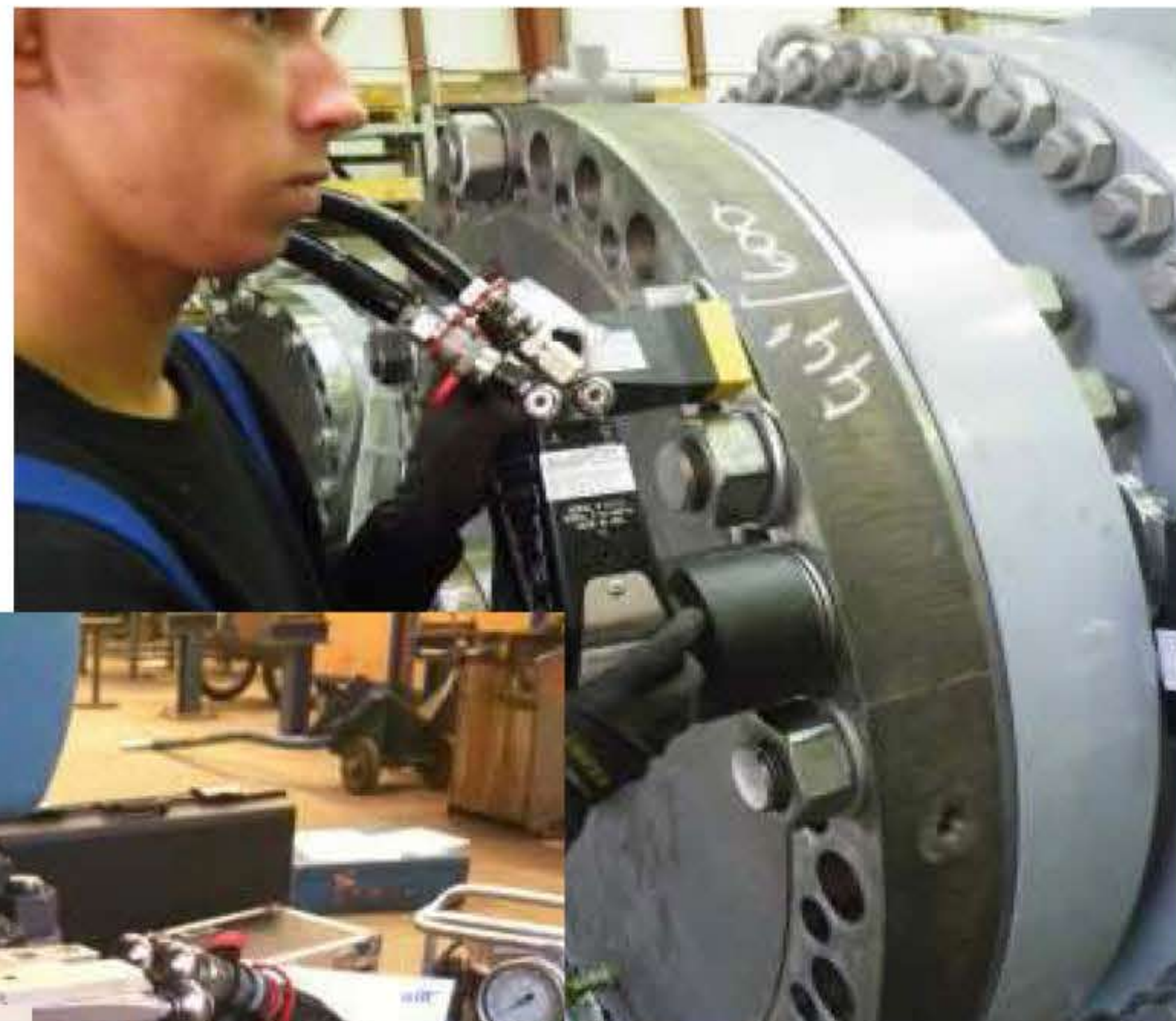
Der RP – Raptor Pneumatik-Drehmomentschrauber bis 8.000 Nm zum Betrieb wie ein Schlagschrauber, aber so genau wie ein Drehmomentschlüssel und viel leiser. Geeignet für Luftnetze mit nur 5,5 bar Fließdruck.
